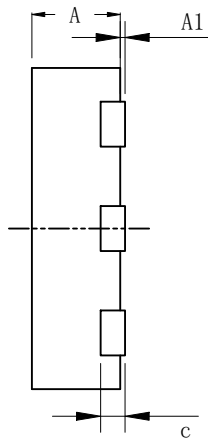
侧视图
