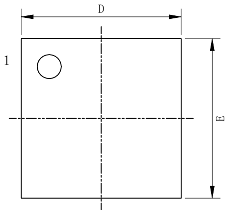
俯视图
